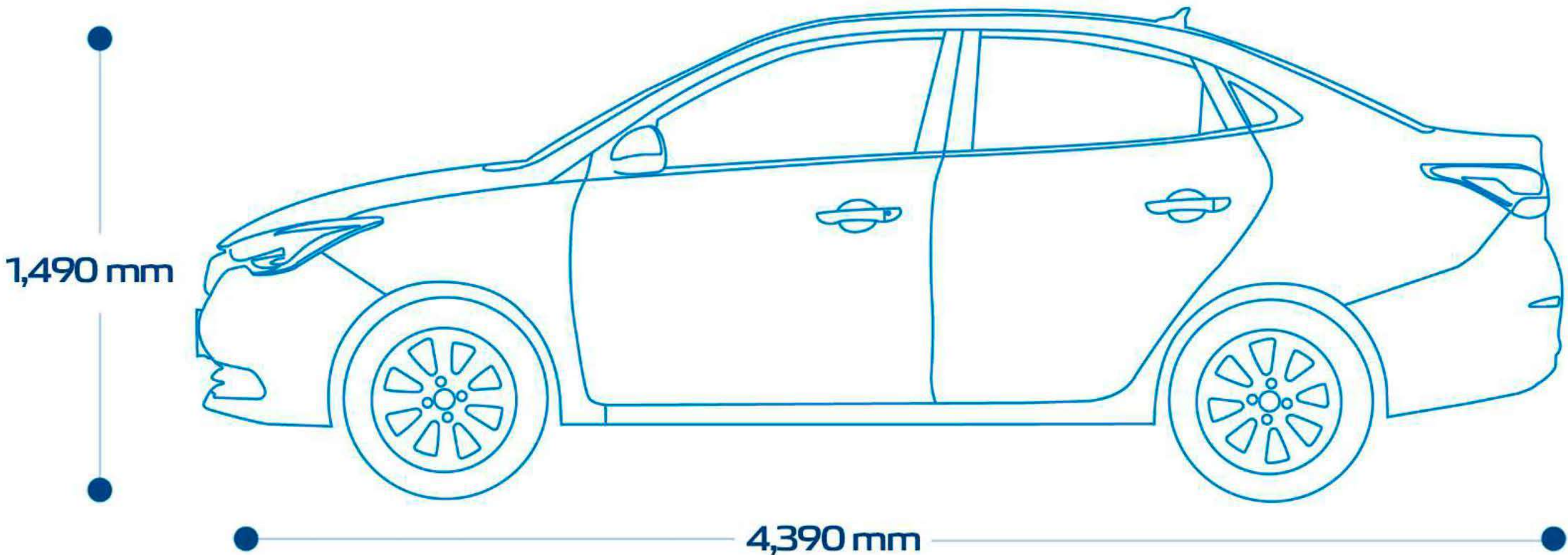
Distancia entre ejes 2,535 mm
